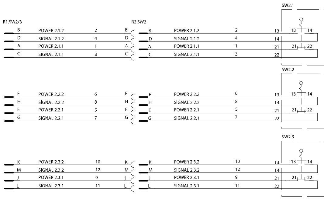
SWITCHES AXIS 2 BRYTARE AXEL 2
